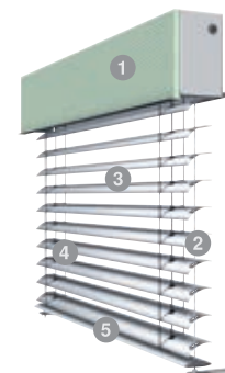
Fenster-System-Außenjalousie E mit sichtbarer Blende und Seilführung
