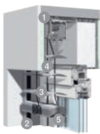
Unterputzausführung
