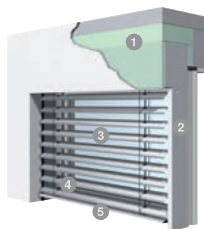
Fenster-System-Außenjalousie P mit Blende in Unterputzausführung
