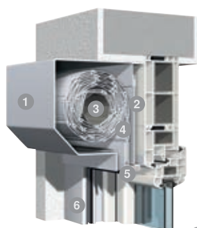
Kastenform Eckig
